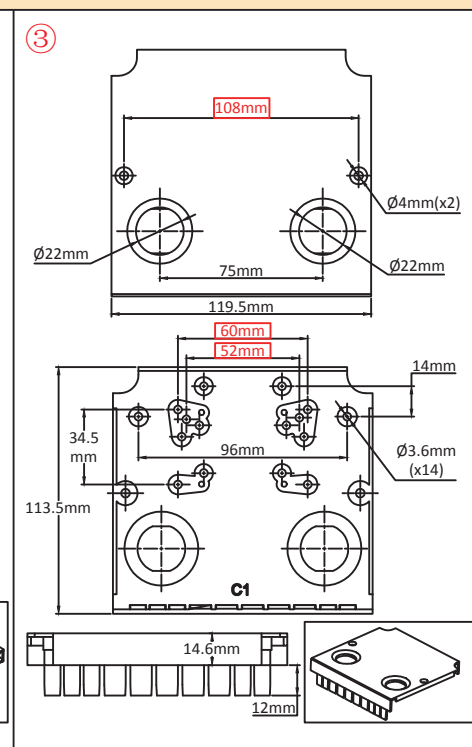
PA66, 两个孔用于 22mm 的指示灯, 一个孔用于保险丝安装托架。螺栓用于继电器
