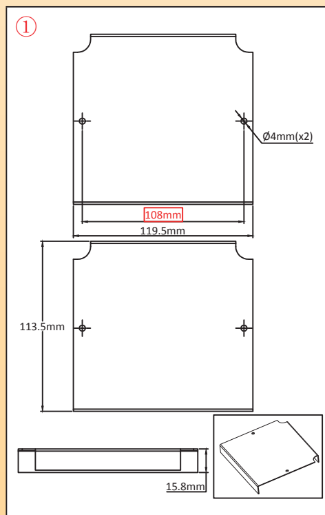
用于客户钻孔和安装的铝板
