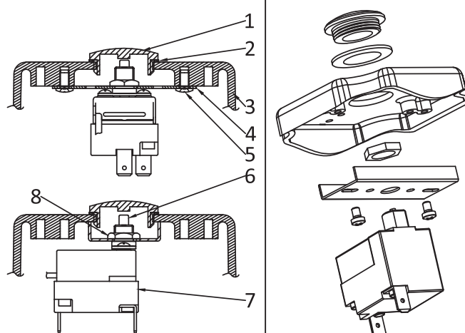
手动复位限制器，在拧紧的帽盖下进入
