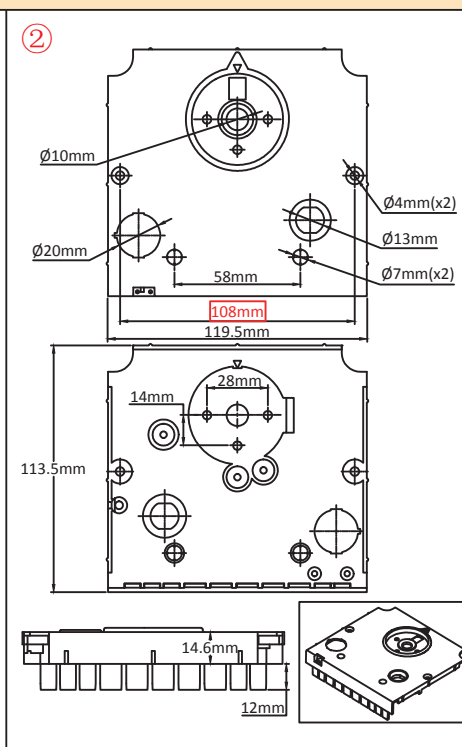
PA66, 用于温控器, 带用于保险丝安装托架的孔, 打开 - 闭合开关和两个指示灯。没有用于继电器的螺栓。
